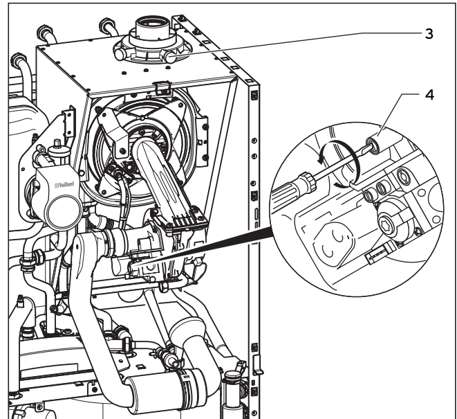
Рис. 6.5 Проверка CO 2
