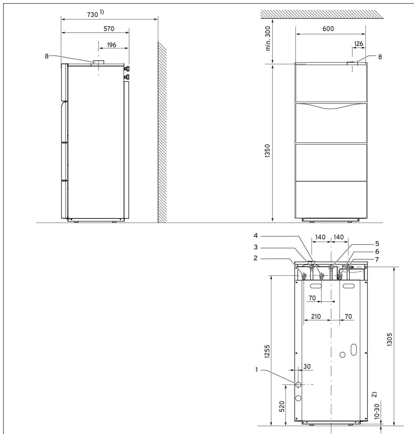
Рис. 4.7 Размеры в мм VSC INT 196/2-С 150 Н, VSC INT 246/2-С 170 Н, VSC INT 306/2-С 200 Н
