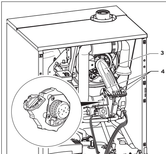
Рис. 9.2 Замена вентилятора
