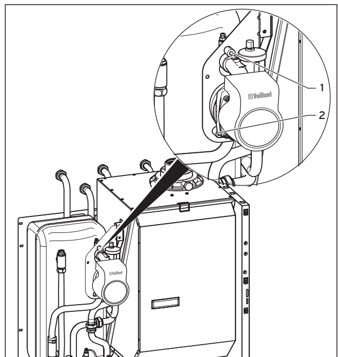
Рис. 8.11 Демонтаж отопительного насоса
