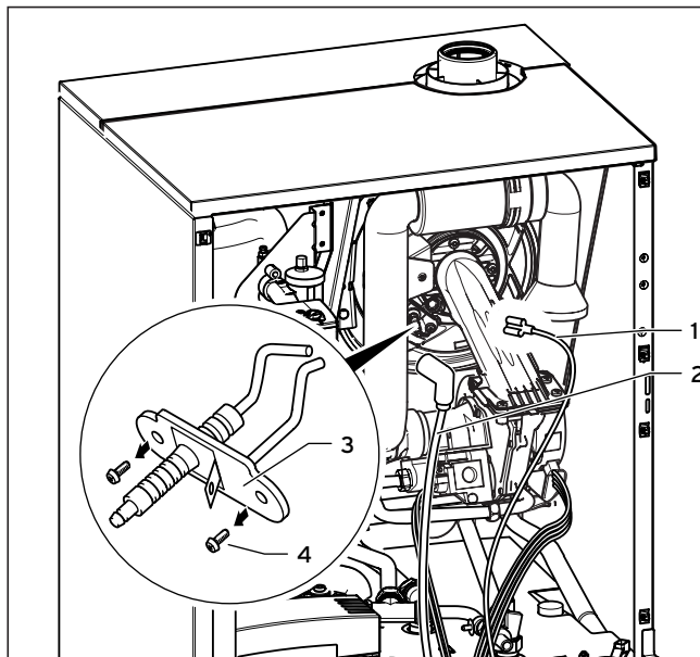
Рис. 9.1 Замена электродов
