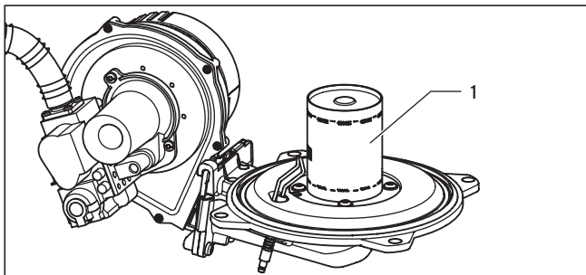
Рис. 8.5 Проверка горелки
